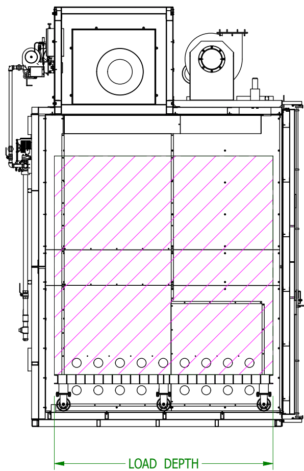
SECTION A-A
